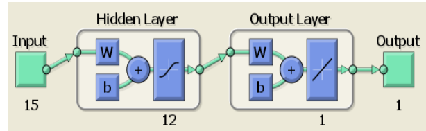
شکل ۵- شبکه عصبی طراحی شده برای تخمین عرض تخم مرغ.
